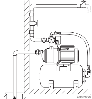
Fig. 2 Funzionamento in aspirazione Suction lift operation Saugbetrieb Fonctionnement en aspiration Funcionamiento en aspiración Sugande funktion Zuigsituatie Θέση λειτουργίας με κάθete αναρρόφηση Работа выше уровня жидкости 负压水头工作
